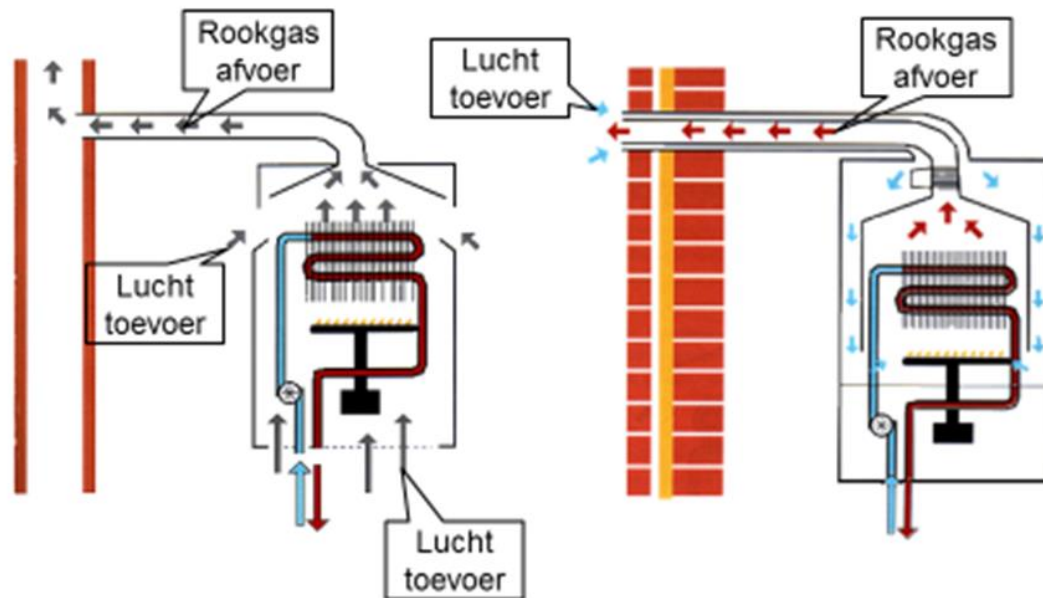
Een open ketel (links) en een gesloten ketel (rechts).
